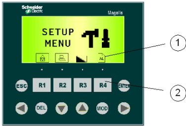
链接到图符的动态功能键的示例
